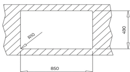
Encastre
