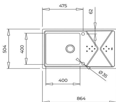
Encastre
