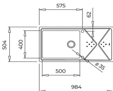
Encastre
