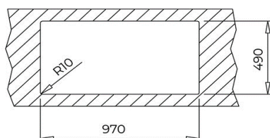
Encastre
